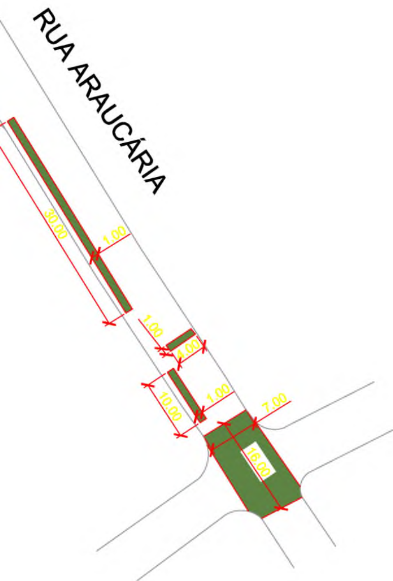
PLANTA BAIXA - REPARO DE BASE SEM ESCALA
